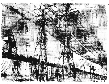
NA BUDOWIE KUBYSZEWSKIEJ ELEKTROWNI WODNEJ. Na zdjęciu: Trasa wiszącej kolekcji linowej na odcinku budowy tamy przelewowej. Fot.—CAF
