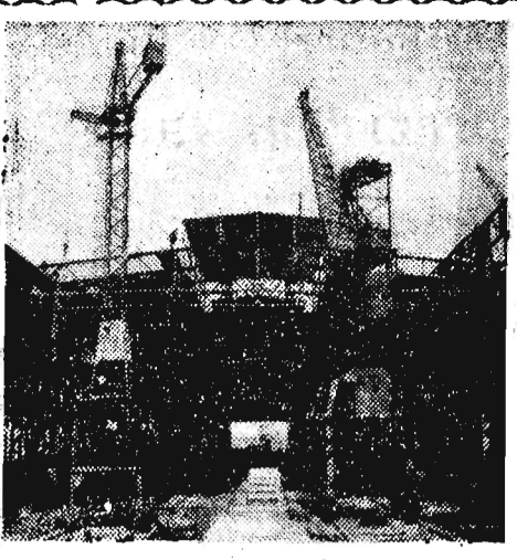
BUDOWA WAŁCOWNI BLACH NA ZIMNO W hucie im. Lenina postępują prace montażowe przy budowie wałcowni blach na zimno. Sześciopiętrowa wałcownia będzie największą halą w Polsce. Będzie produkować 400 tys. ton blachy rocznie o grubości od 2,5 milimetra do 0,24 mm. Na zdjęciu: Fragment budowy wałcowni. CAF — fot. Link.
