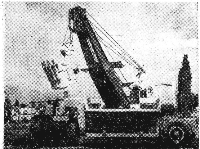
Na zdjęciu: Uniwersalna koparka czeskosłowacka E-25. Pojemność czepaka — 2,5 m 3 , wystawiona na Trzecich Targach Technicznych w Brnie. Fot — CAF
