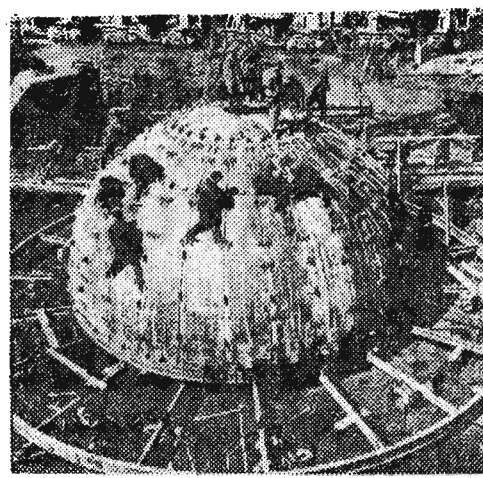
Na budowie nowego wielkiego pieca w Kuźnieckim Kombi-nacie Metalurgicznym w Stalińsku wkrótce zakończą się prace betoniarzkie. Na zdjęciu: Montaż kopuły wielkiego pieca.
