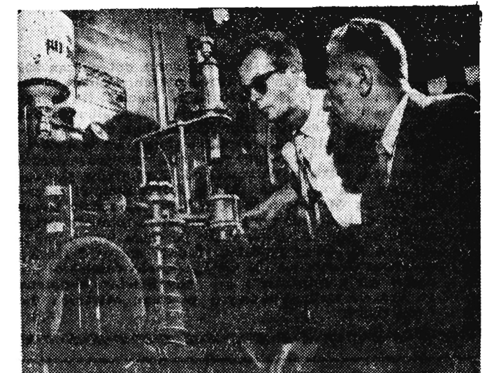
Pracownicy naukowcy laboratorium Instytutu Radioelektroniki i Elektroniki; profesor doktor S. Katalanow i kandydat nauk fizyko-matematycznych J. Pokrowski są twórcami oryginalnej metody otrzymywania chemicznie czystego krzemu. CAF
