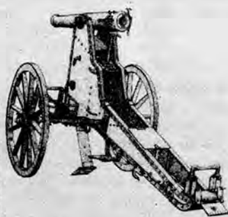
Armaty kal. 9 cm wz. M.75 znaleziona w Siedliskach, umieszczona była na tzw. wysokiej, kazonowej lawecie. Zainstalowana w lewej kaponierze fortu służyła do obrony fosy. Przystosowana była do strzału granatem (donośność 6,5 km), do strzału szrapnelem lub do strzału kartaczem (donośność 400 m).
