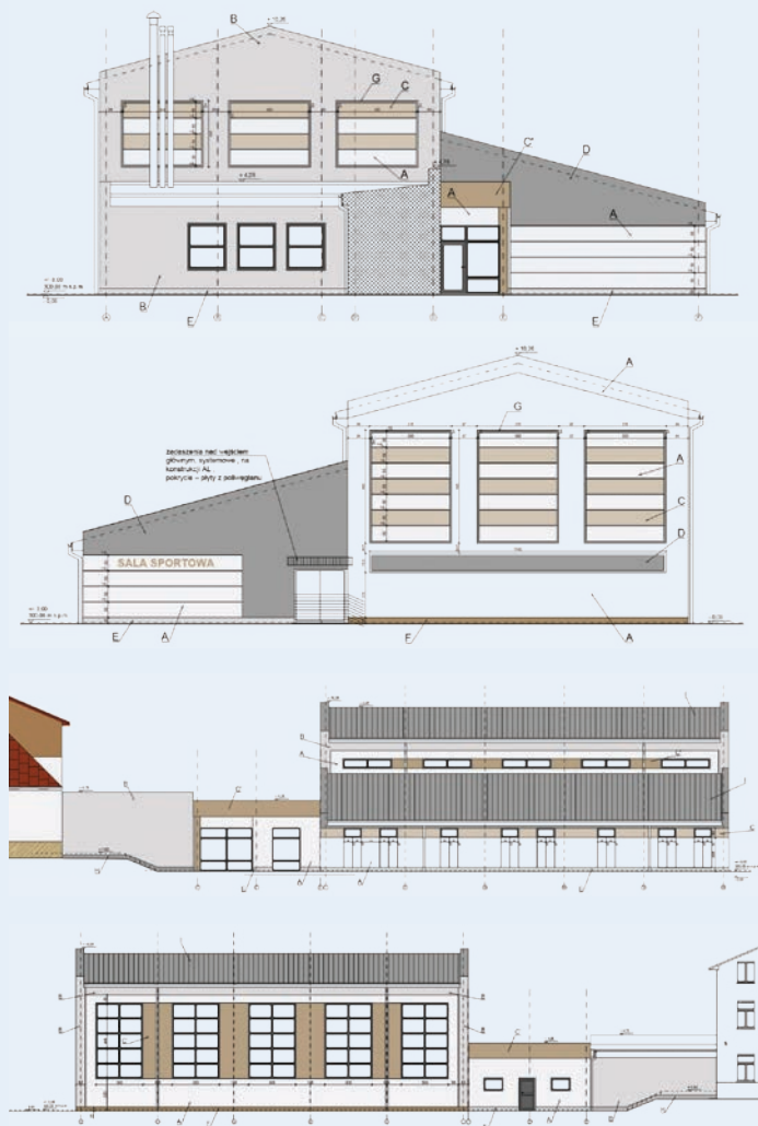
Projekt sali gimnastycznej przy szkole w Zalesiu (Biuro Usług Projektowych i Inwestycyjnych „Dominex”)
