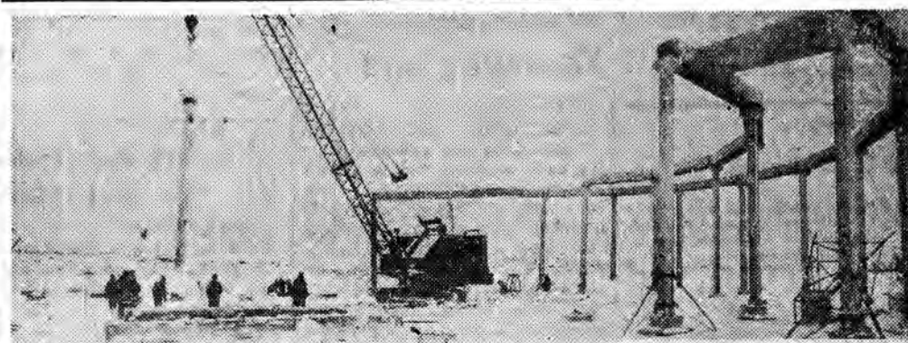
Budowa olbrzymich żelazobetonowych zbiorników na ropę naftową w obwodzie Kujbyszewskim, skąd będzie ona odprowadzana rurociągiem „Puzgłak”. Na zdjęciu: montaż kolumny podtrzymujących zbiorniki. CAF
