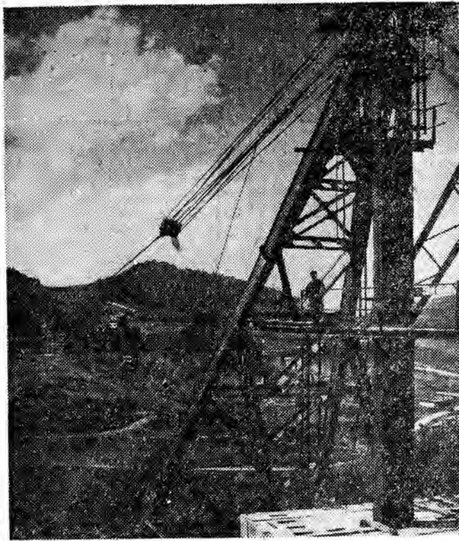
Budowa Zapory Wodnej na Sanie w Solinie rozpoczęła się w 1960 r. Uruchomienie pierwszego turbozespołu ma nastąpić w IV kwartale 1966 r., natomiast II, III i IV zostaną oddane do użytku do grudnia 1967 r.
