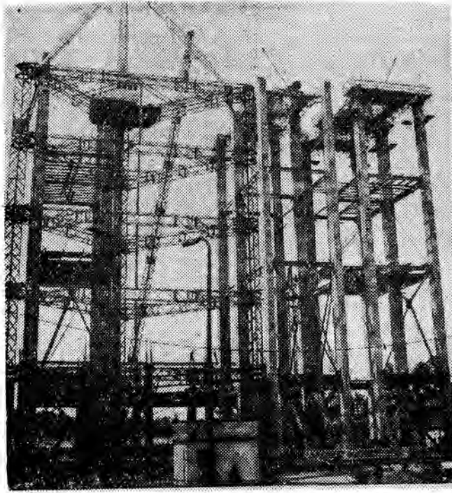
ROZBUDOWA ELEKTROWNI W STALOWEJ WOLI Trwają prace przy wznoszeniu nowych obiektów Elektrowni w Stalowej Woli, które dzięki zastosowaniu nowych metod budowlanych zostaną w stanie surowym ukończone jeszcze w tym roku. Po uruchomieniu nowego obiektu moc Elektrowni Stalowa Wola wzrośnie o dalszych 250 MW. Na zdjęciu: Prace budowlane i montażowe. CAF — fot. Kwiatkowski
