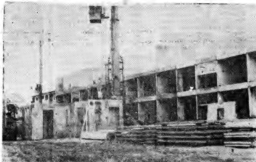
Montaż domów z prefabrykatów. Jeden dźwig, kilku robotników, ustawiających we właściwym miejscu elementy, a to cała tajemnica powodzenia i procesu budowy.
